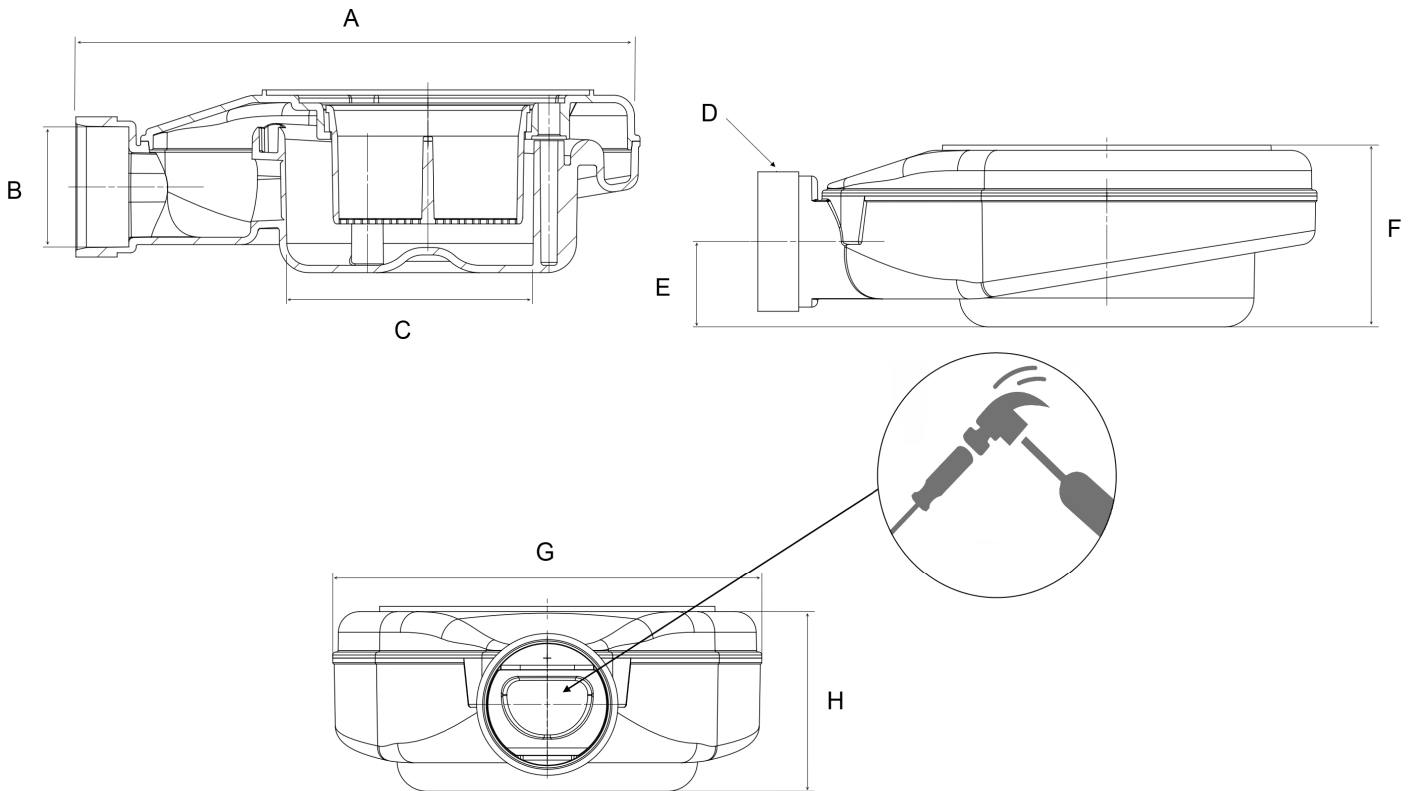
Cotas (mm)
